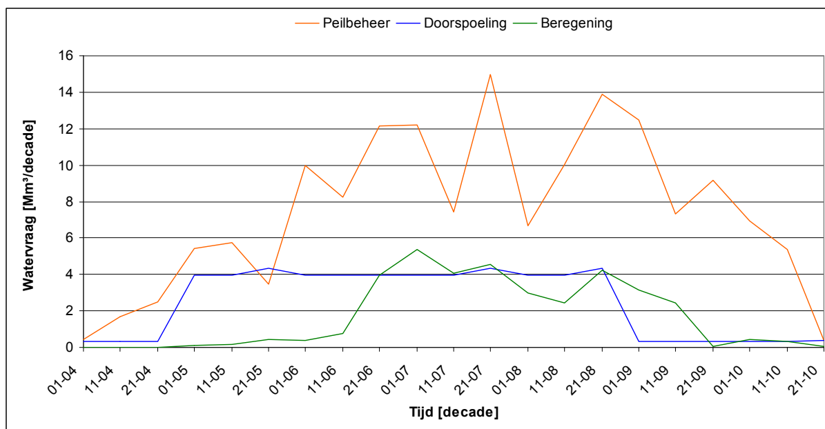
Figuur 6.3: Watervraag per functie tijdens het zomerhalfjaar voor het jaar 1949 onder klimaatscenario G+ en extra berekeningareaal in 2100.
