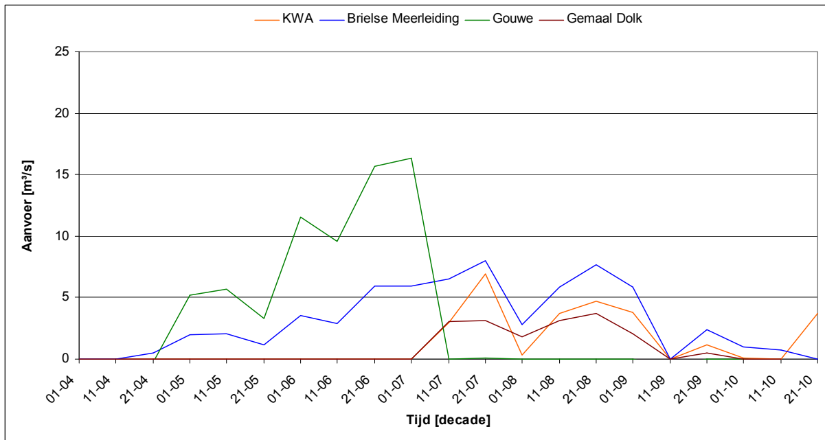
Figuur 8.8: Debiet in de aanvoerroutes de Gouwe, KWA, Brielse Meerleiding en gemaal Dolk tijdens het zomerhalfjaar voor het jaar 1949 onder klimaatscenario G+ en extra beregeningsareaal in 2050.
