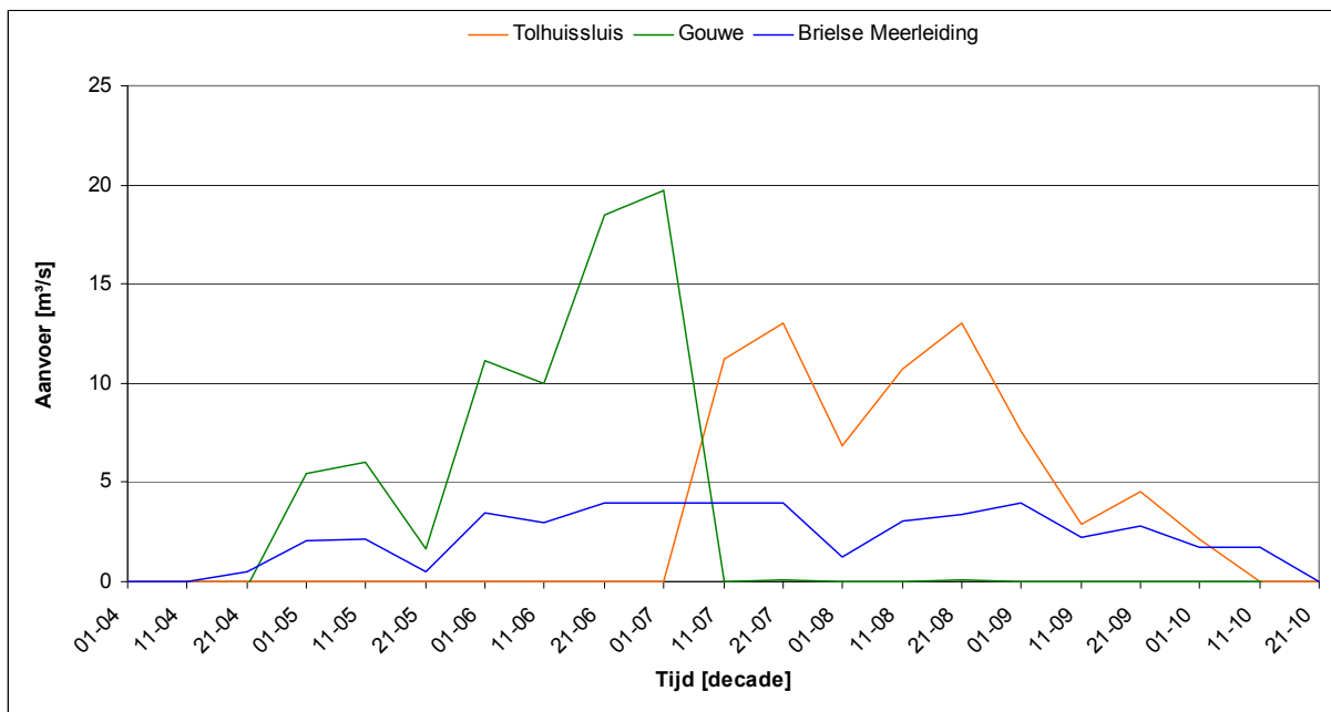
Figuur 8.6: Debiet in de aanvoerroutes de Gouwe, Tolhuissluis en Brielse Meerleiding tijdens het zomerhalfjaar voor het jaar 1949 onder klimaatscenario G+ en extra beregeningsareaal in 2100 [m³/s].
