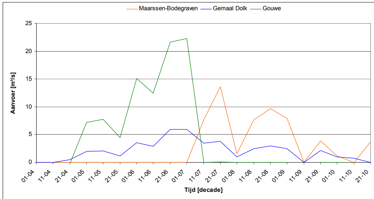
Figuur 8.10: Debiet in de aanvoerroutes de Gouwe, gemaal Dolk en Maarssen-Bodegraven tijdens het zomerhalfjaar voor het jaar 1949 onder klimaatscenario G+ en extra beregeningsareaal in 2050 [m³/s].
