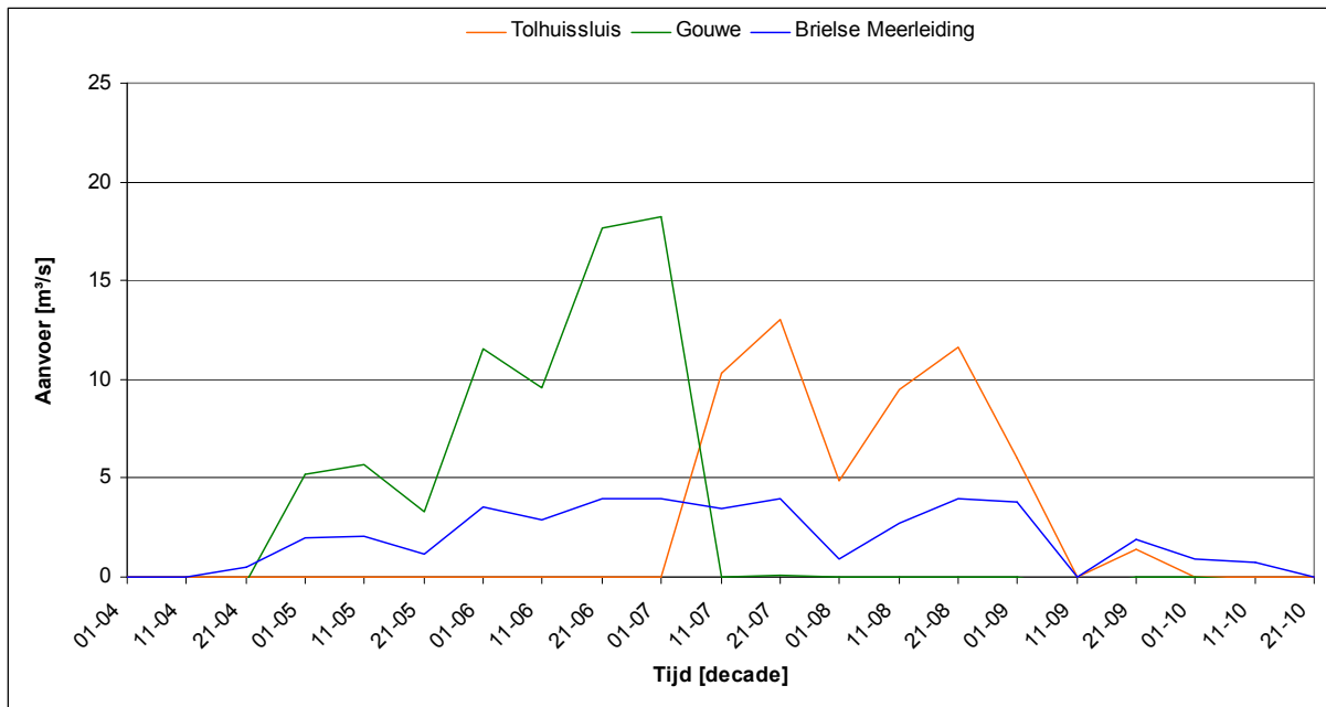
Figuur 8.5: Debiet in de aanvoerroutes de Gouwe, Tolhuissluis en Brielse Meerleiding tijdens het zomerhalfjaar voor het jaar 1949 onder klimaatscenario G+ en extra beregeningsareaal in 2050 [m³/s].
