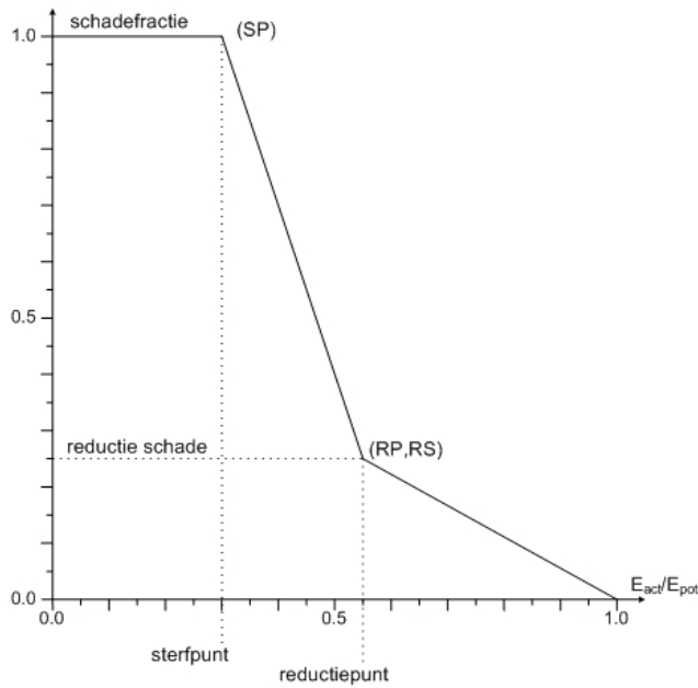
Figuur B.3: Grafisch weergave van de functie voor verdrassingsschade (bron: Mulder et al. (2010)). Waarin: E_{act} = actuele verdamping [mm], E_{pot} = potentiële verdamping [mm], RP= reductiepunt [-], RS= reductieschade [-] en SP= sterfpunt [-].
