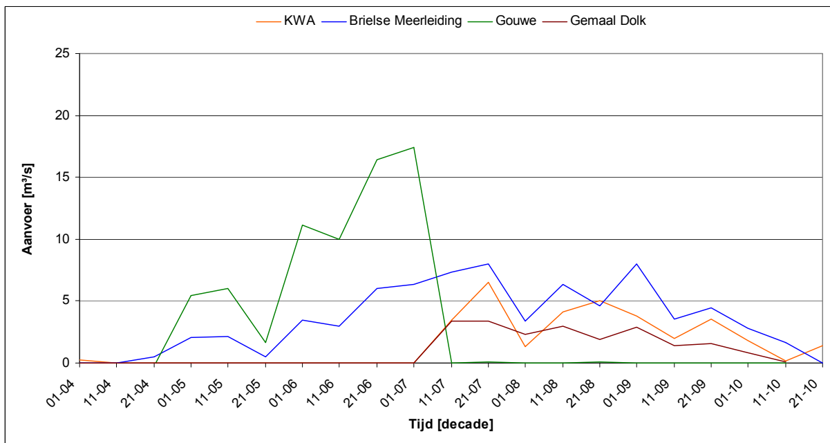
Figuur 8.9: Debiet in de aanvoerroutes de Gouwe, KWA, Brielse Meerleiding en gemaal Dolk tijdens het zomerhalfjaar voor het jaar 1949 onder klimaatscenario G+ en extra beregeningsareaal in 2100.
