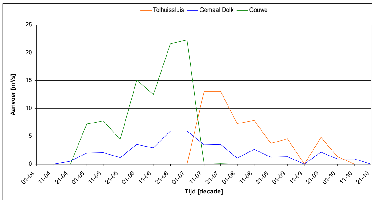
Figuur 8.3: Debiet in de aanvoerroutes de Gouwe, gemaal Dolk en Tolhuissluis tijdens het zomerhalfjaar voor het jaar 1949 onder klimaatscenario G+ en extra beregeningsareaal in 2050 [m³/s].
