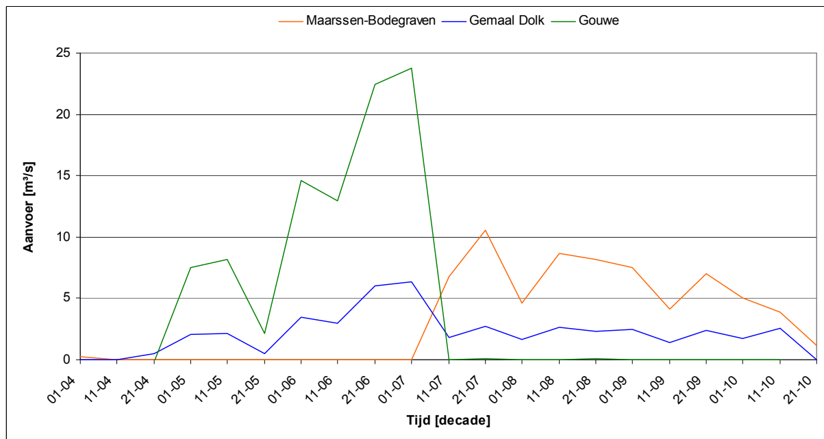
Figuur 8.11: Debiet in de aanvoerroutes de Gouwe, gemaal Dolk en Maarssen-Bodegraven tijdens het zomerhalfjaar voor het jaar 1949 onder klimaatscenario G+ en extra beregeningsareaal in 2100 [m³/s].
