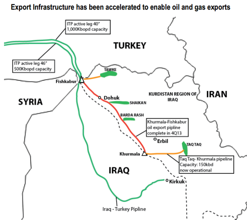
FIGUUR 6 - OLIEPIJPLEIDINGEN IN IRAK EN DE KRG NAAR TURKIJE.
