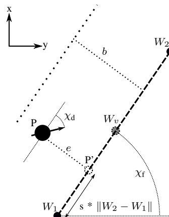
Fig. 1. Control problem parameters
