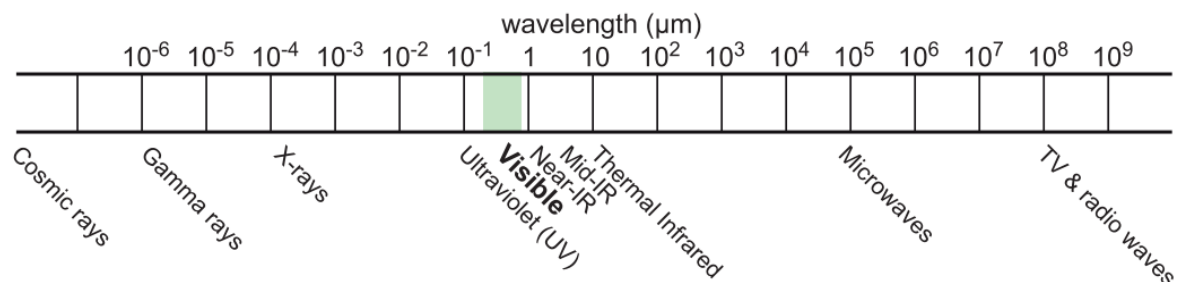
Fig. 8 The classification of EM spectrum (Bakx et al., 2012).
