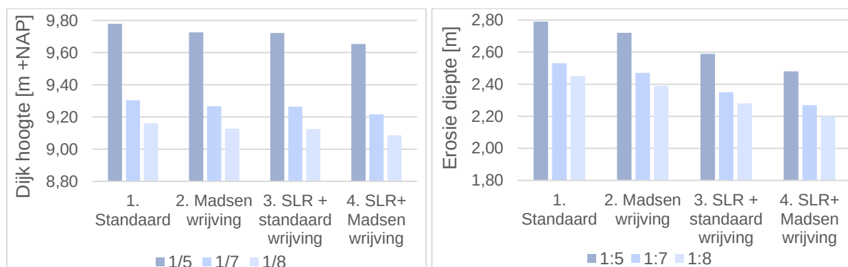
Figuur 2. Benodigde dijkafmetingen voor verschillende scenario's
